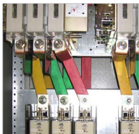
Трубки для цветовой маркировки проводов
