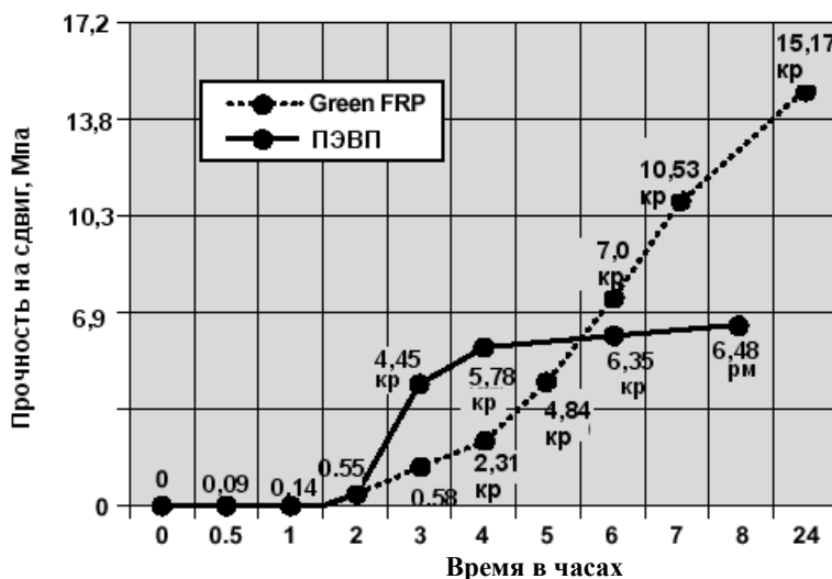
Рис.2 Нарастание прочности со временем.
