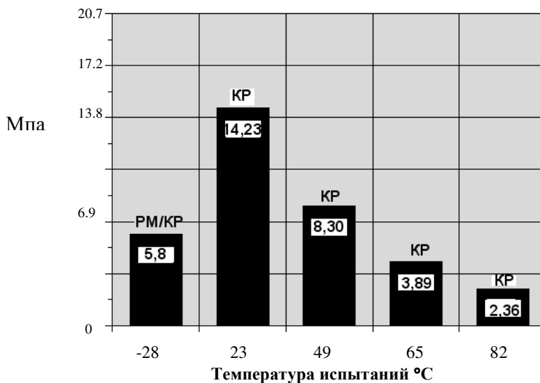
Рис.1 Прочность на сдвиг при различных температурах.
